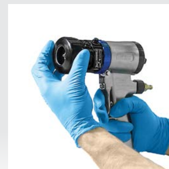
Remplacez le circlip et le chapeau d'air
